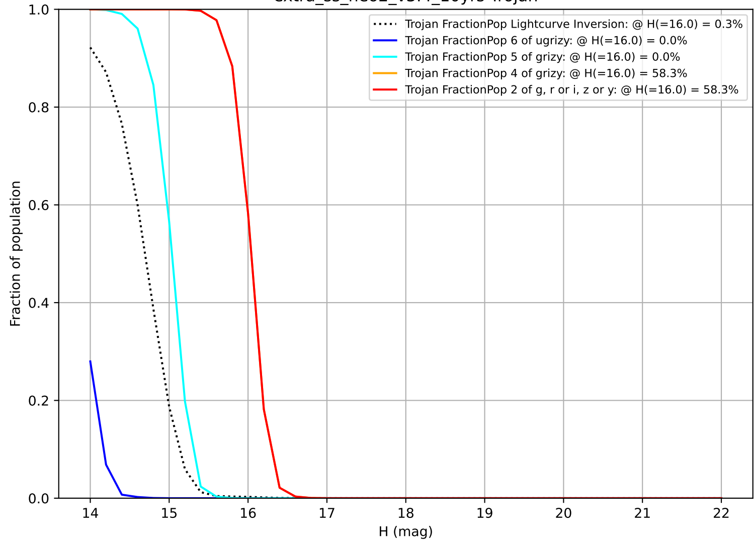
extra_ss_neo2_v3.4_10yrs Trojan
