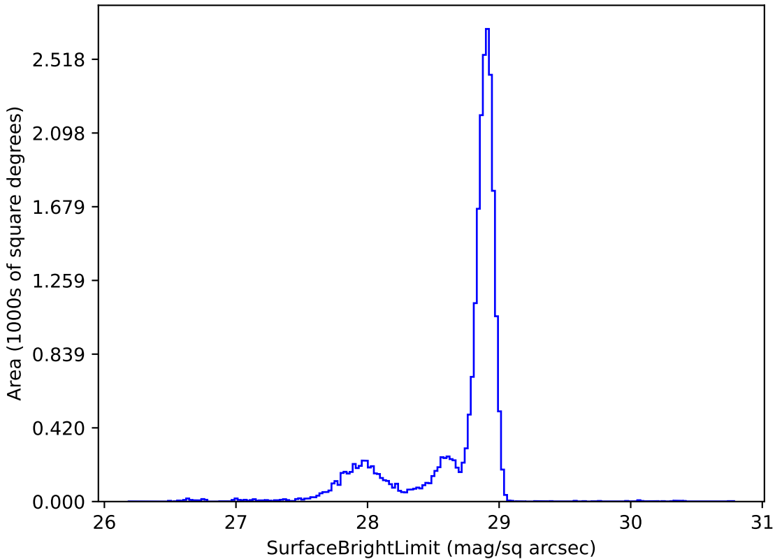
extra_ss_neo2_v3.4_10yrs u: SurfaceBrightLimit
