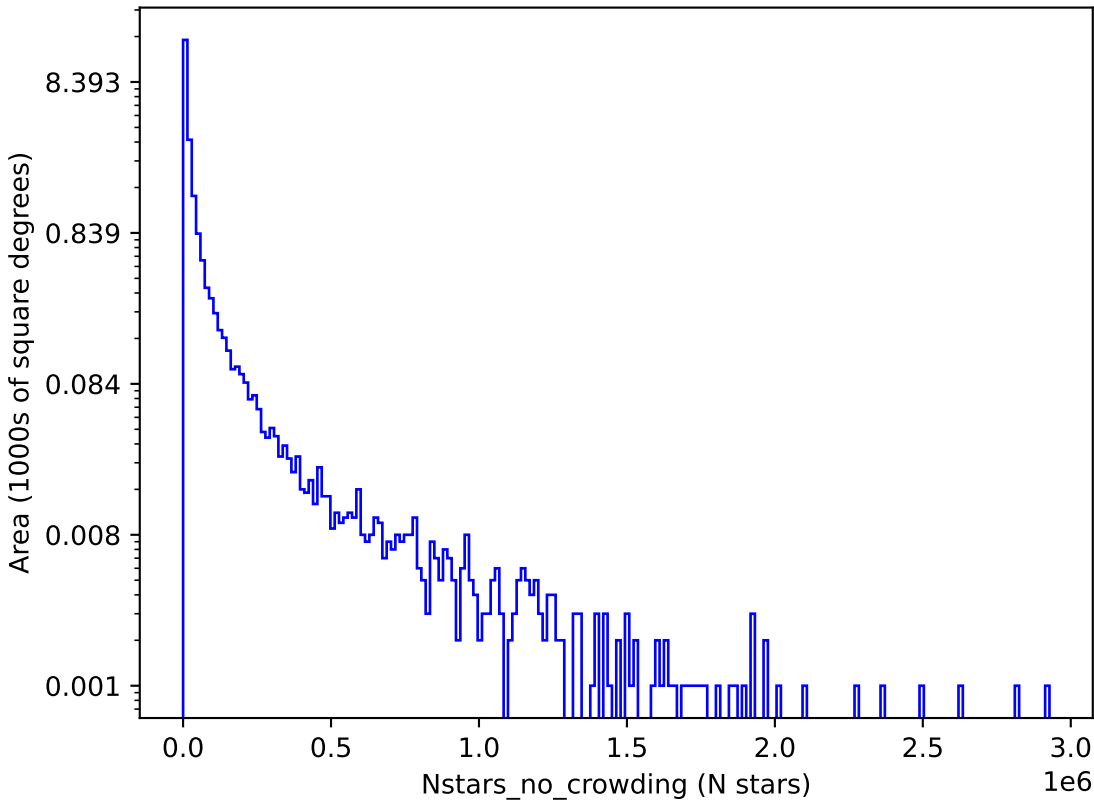
extra_ss_neo2_v3.4_10yrs u: Nstars_no_crowding
