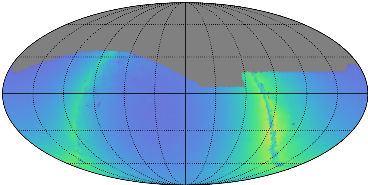
extra_ss_neo2_v3.4_10yrs g: Nstars_no_crowding
