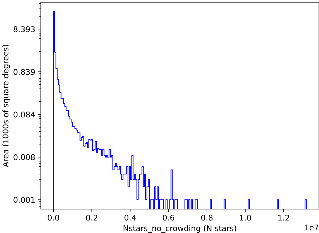
extra_ss_neo2_v3.4_10yrs g: Nstars_no_crowding
