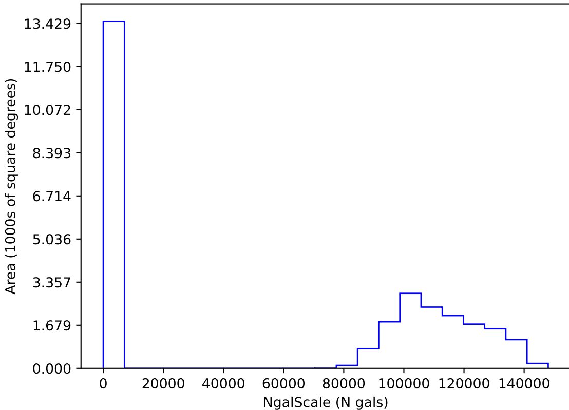
extra_ss_neo2_v3.4_10yrs i: NgalScale
