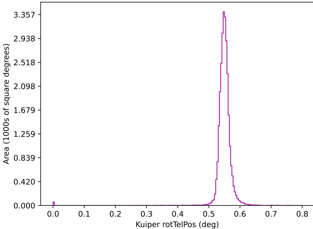
extra_ss_neo2_v3.4_10yrs z: Kuiper rotTelPos
