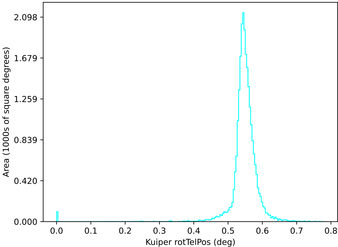
extra_ss_neo2_v3.4_10yrs u: Kuiper rotTelPos
