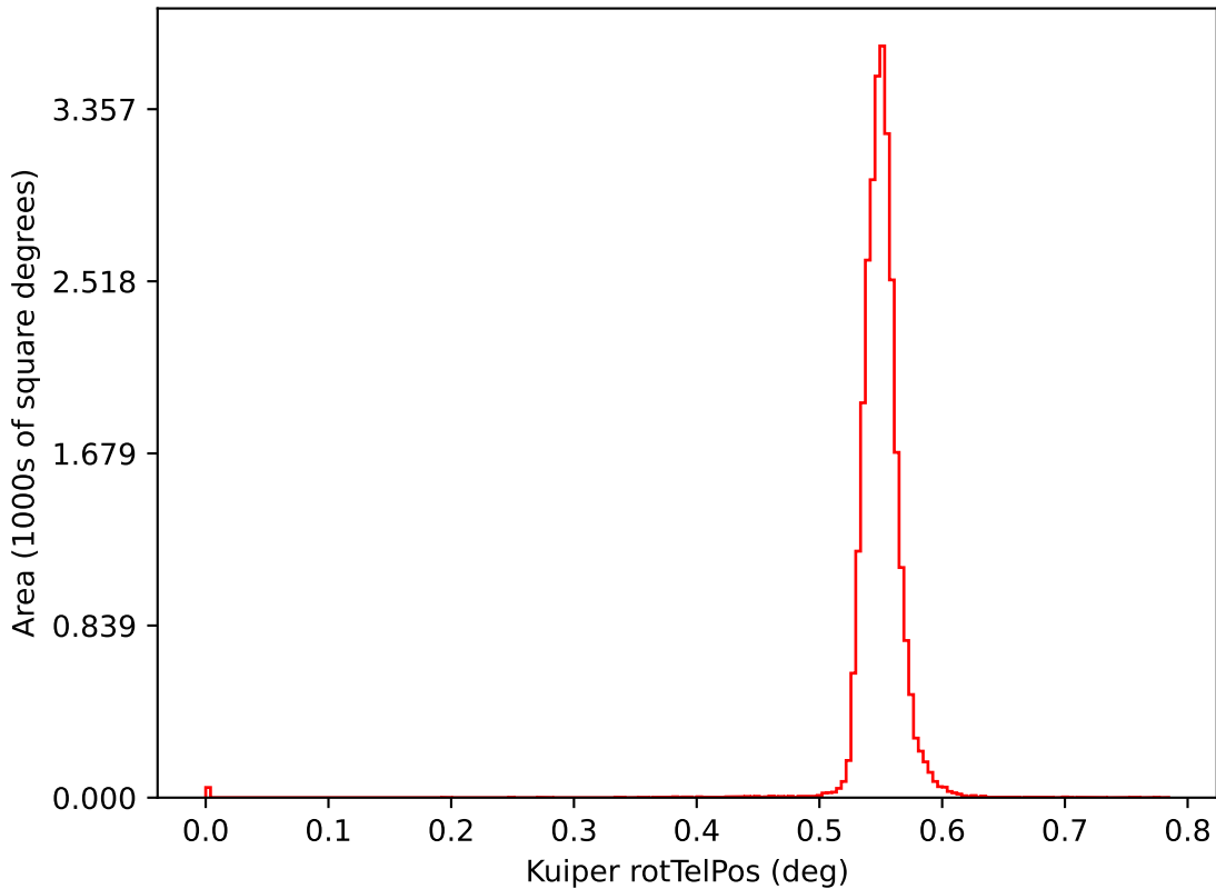
extra_ss_neo2_v3.4_10yrs i: Kuiper rotTelPos
