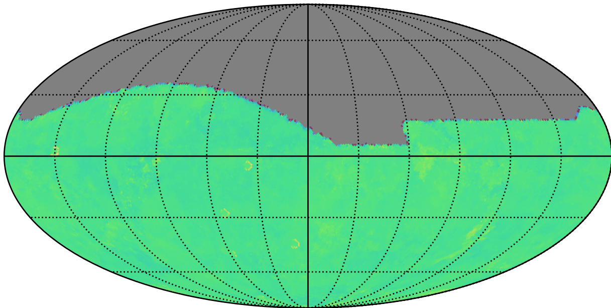
extra_ss_neo2_v3.4_10yrs g: Kuiper rotTelPos
