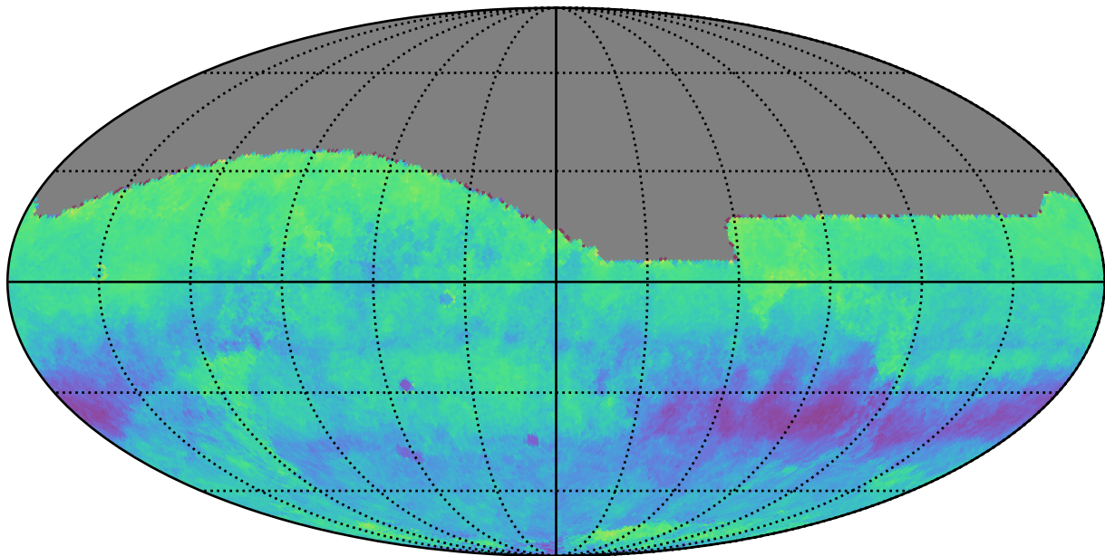
extra_ss_neo2_v3.4_10yrs r: Kuiper rotSkyPos
