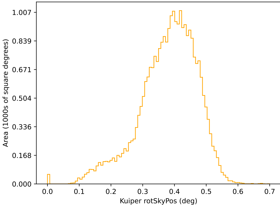
extra_ss_neo2_v3.4_10yrs r: Kuiper rotSkyPos
