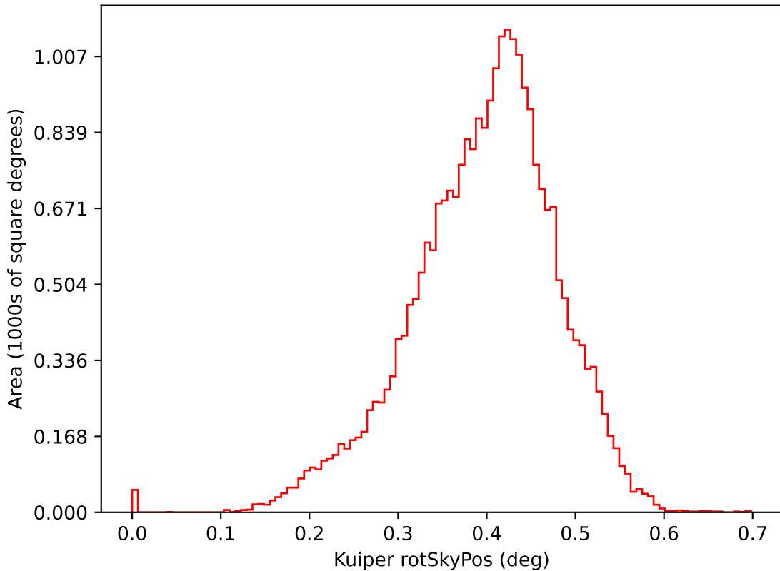
extra_ss_neo2_v3.4_10yrs i: Kuiper rotSkyPos
