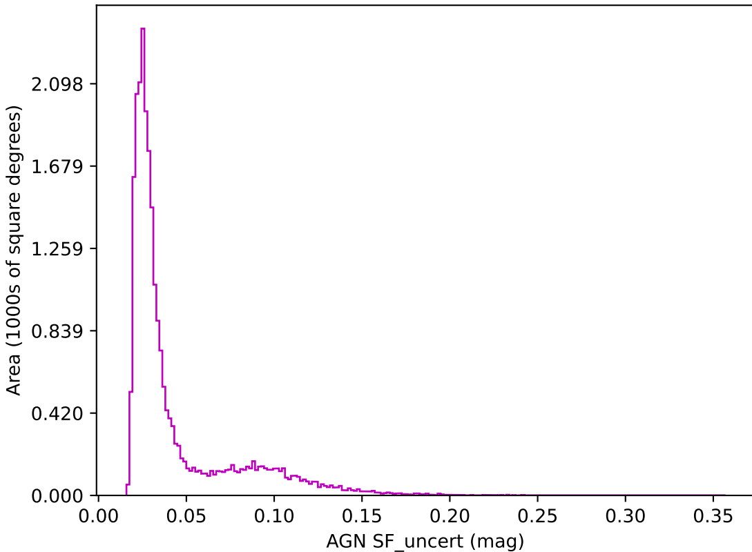
extra_ss_neo2_v3.4_10yrs z band: AGN SF_uncert
