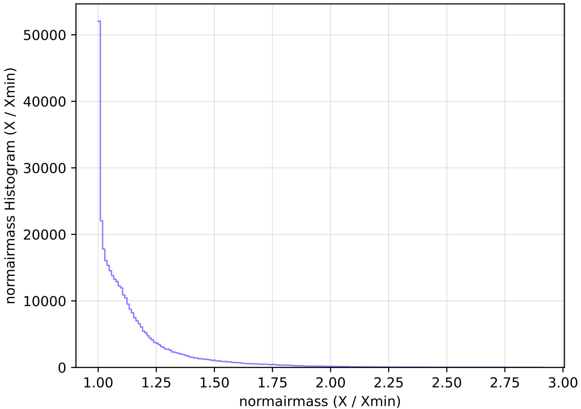
extra_ss_neo2_v3.4_10yrs WFD y band: normairmass Histogram
