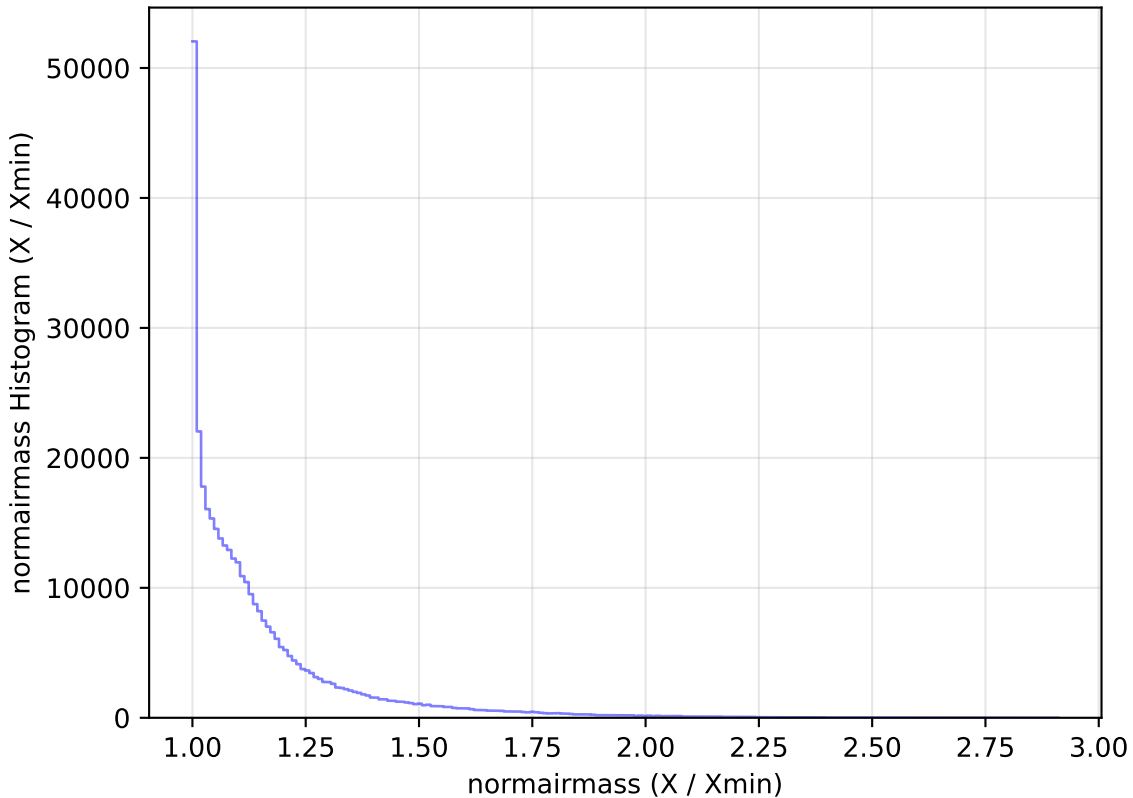
extra_ss_neo2_v3.4_10yrs All sky y band: normairmass Histogram
