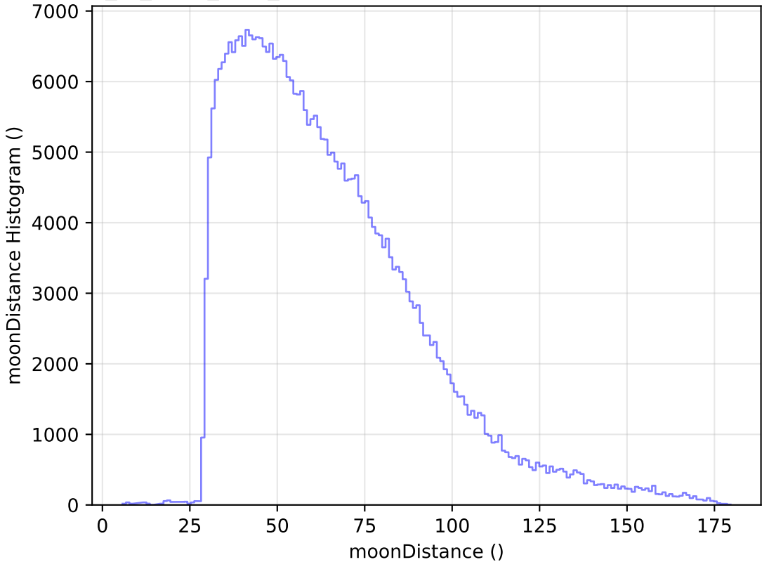
extra_ss_neo2_v3.4_10yrs All sky y band: moonDistance Histogram
