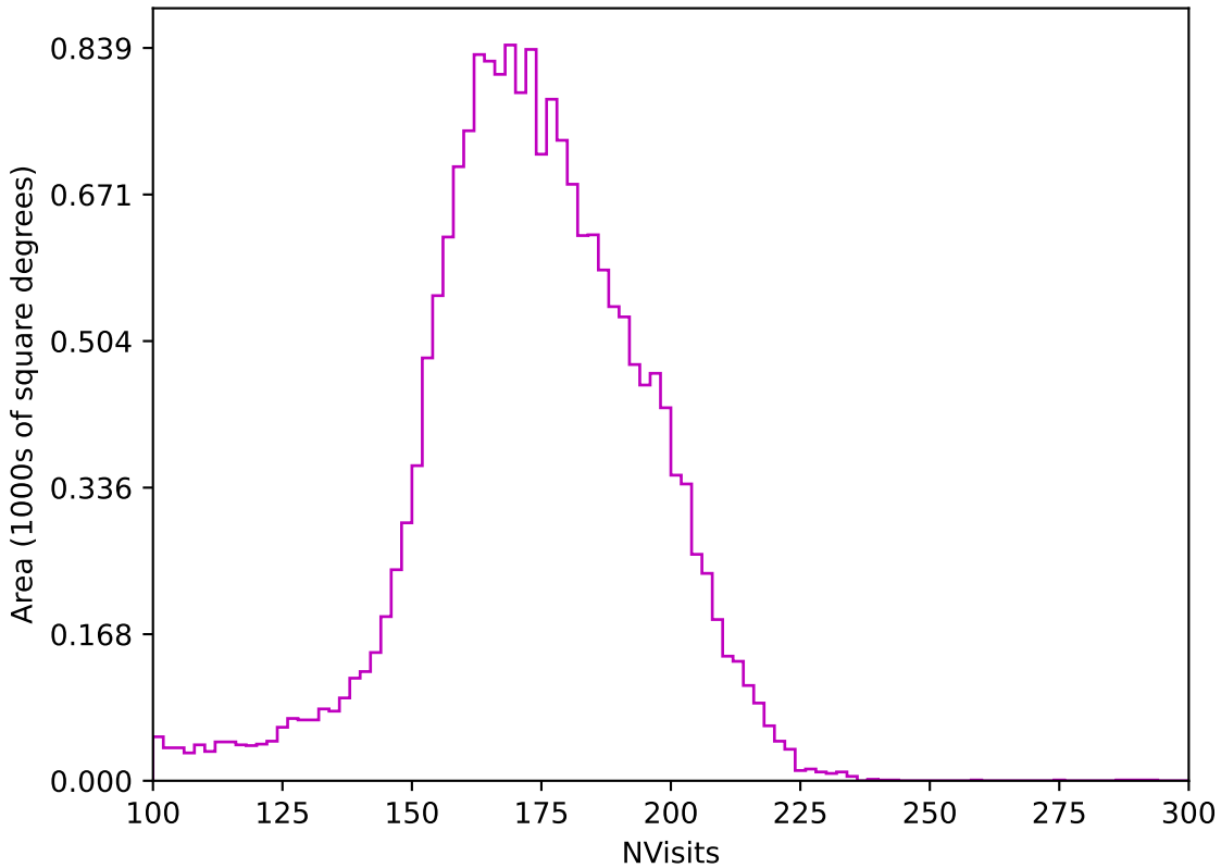
extra_ss_neo2_v3.4_10yrs All sky z band: NVisits
