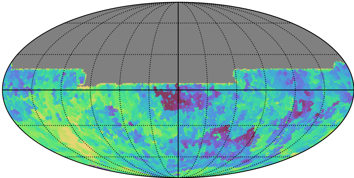
extra_ss_neo2_v3.4_10yrs All sky y band: Min saturation_mag
