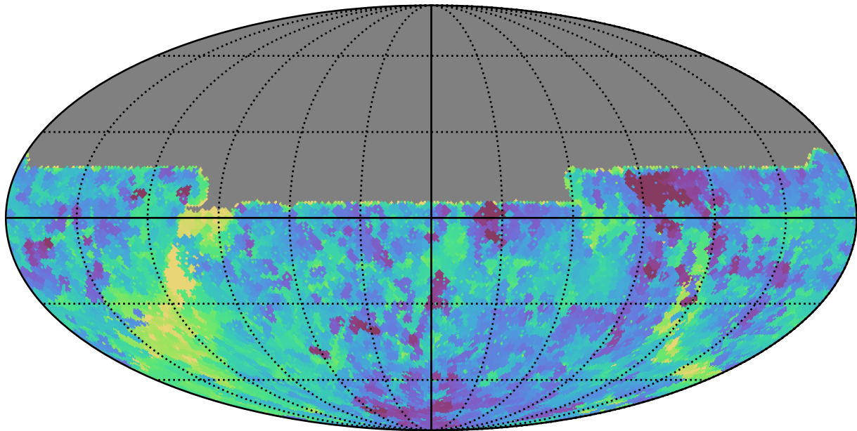
extra_ss_neo2_v3.4_10yrs All sky u band: Min saturation_mag
