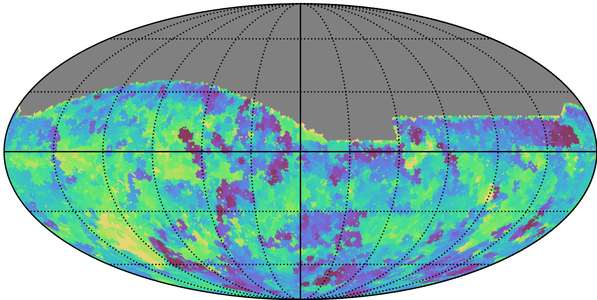
extra_ss_neo2_v3.4_10yrs All sky g band: Min saturation_mag
