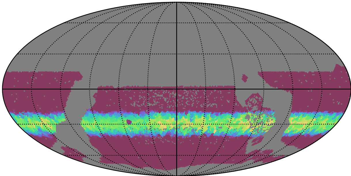
extra_ss_neo2_v3.4_10yrs WFD z band: Min normairmass
