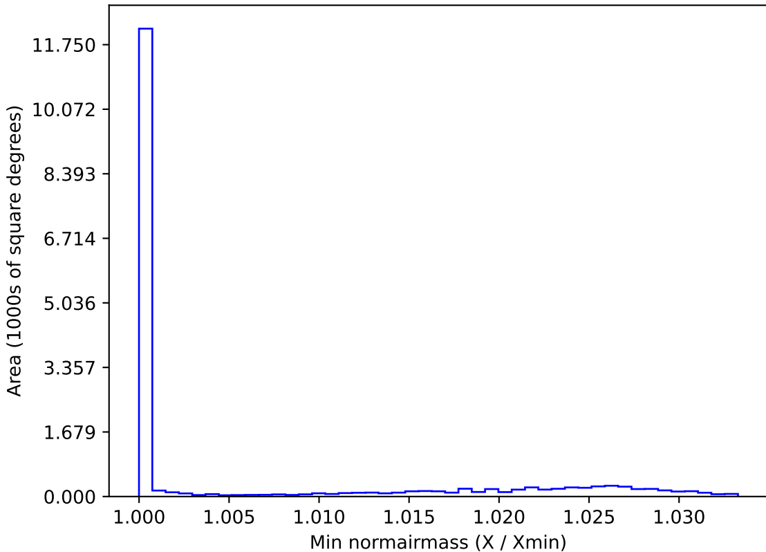
extra_ss_neo2_v3.4_10yrs WFD z band: Min normairmass
