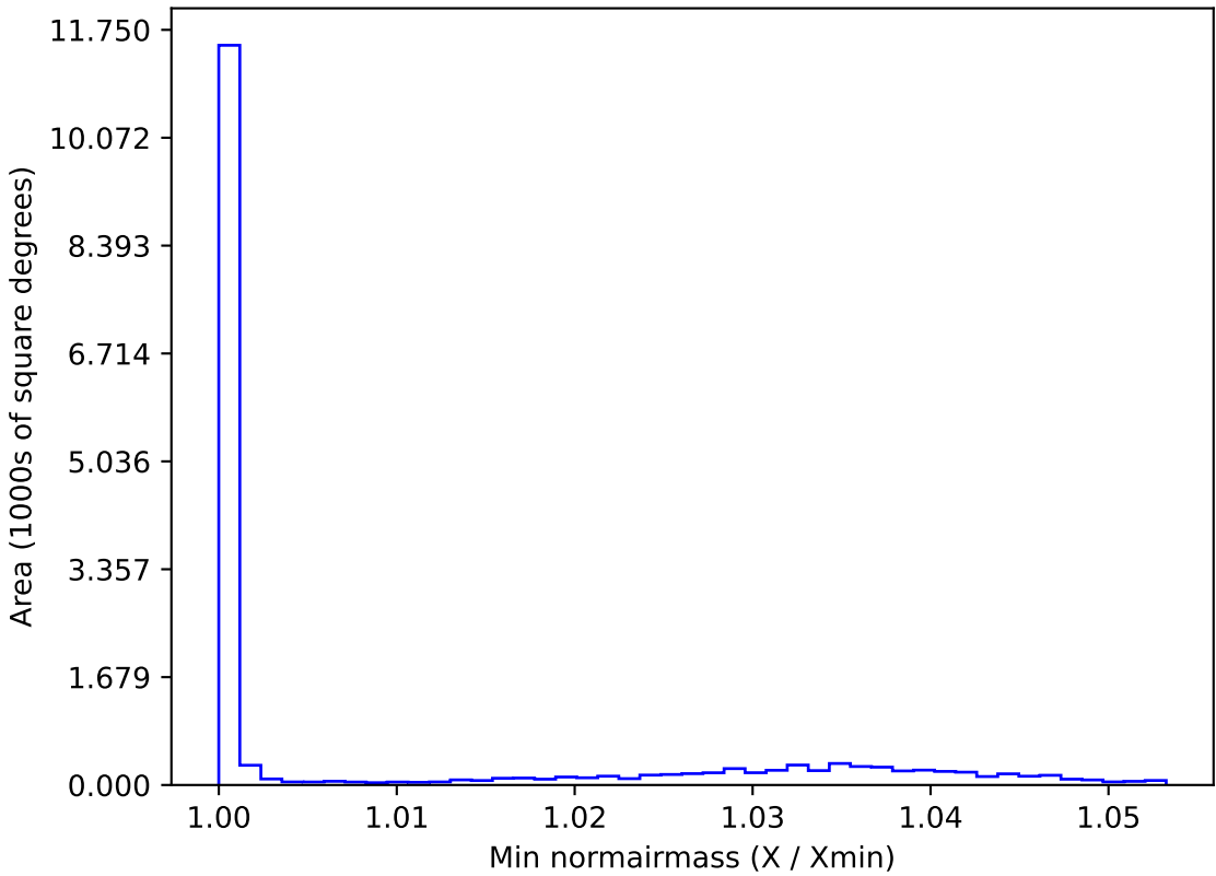
extra_ss_neo2_v3.4_10yrs WFD u band: Min normairmass
