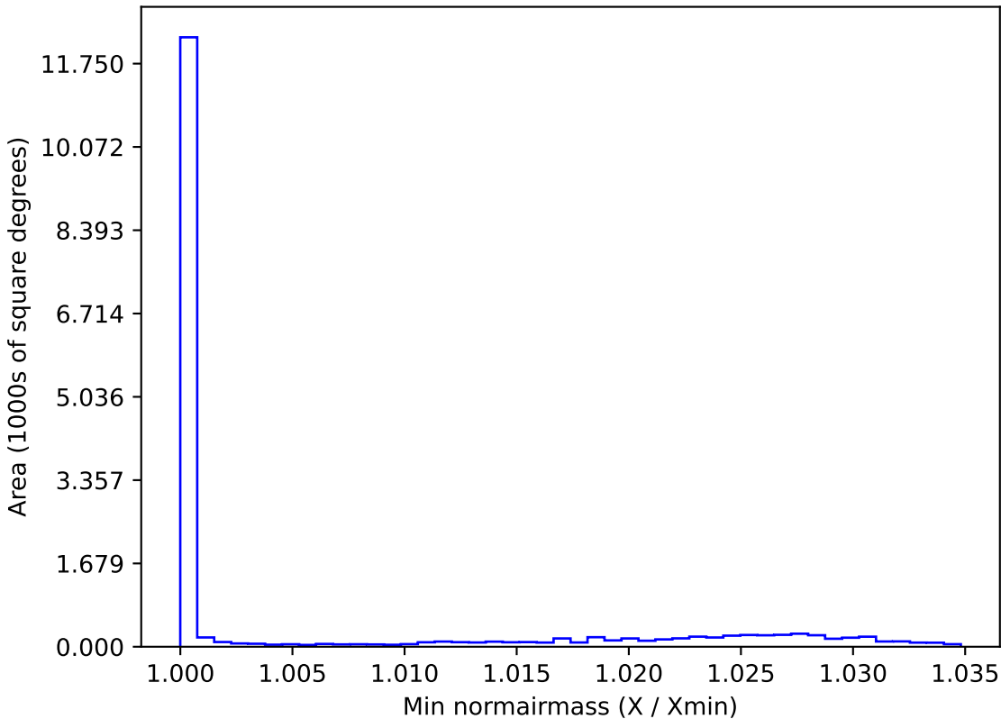
extra_ss_neo2_v3.4_10yrs WFD i band: Min normairmass
