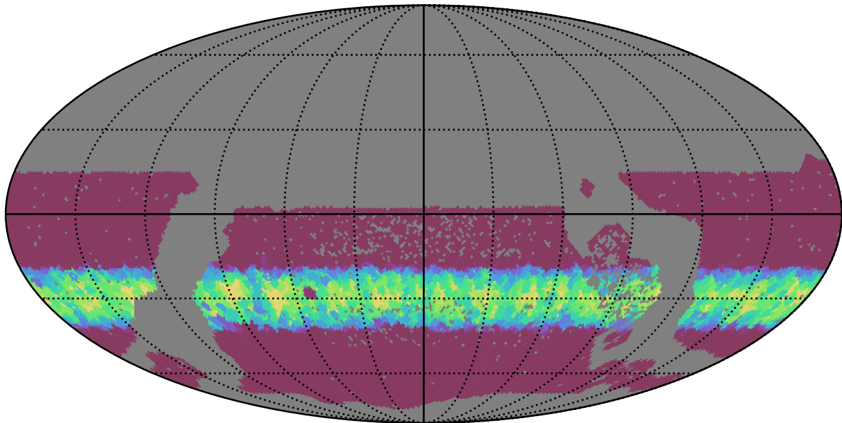
extra_ss_neo2_v3.4_10yrs WFD g band: Min normairmass
