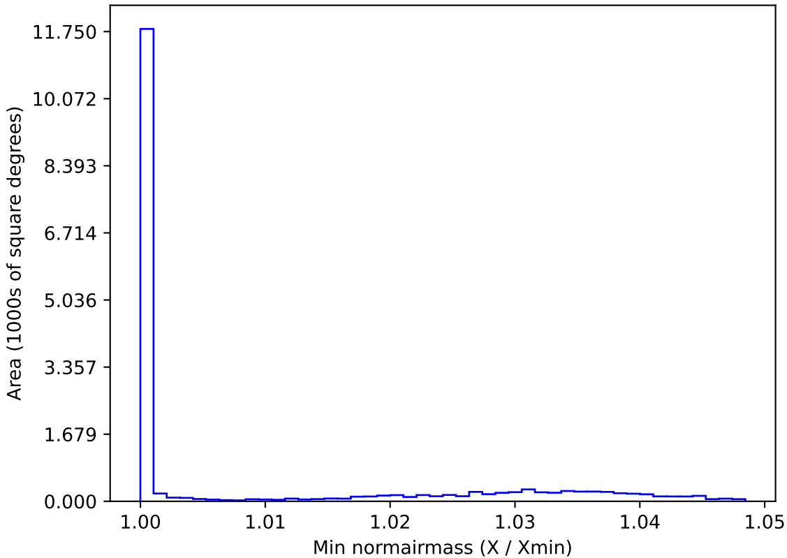
extra_ss_neo2_v3.4_10yrs WFD g band: Min normairmass
