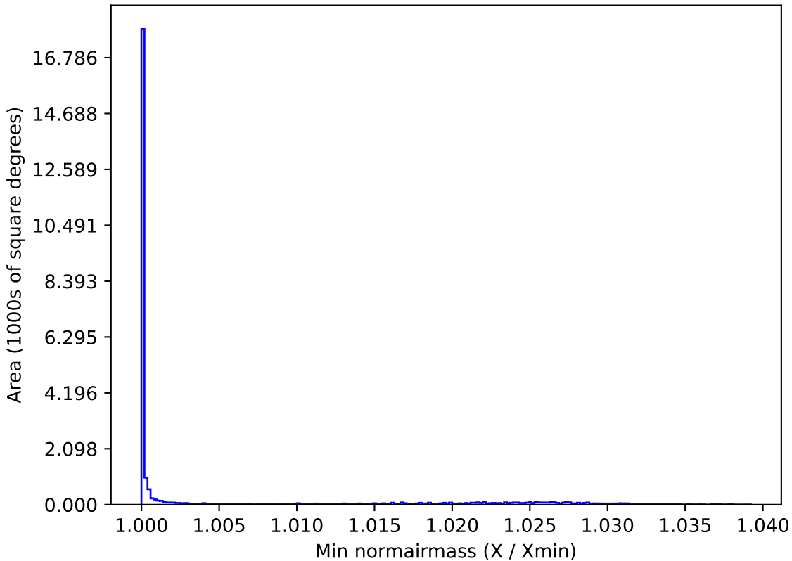
extra_ss_neo2_v3.4_10yrs All sky z band: Min normairmass
