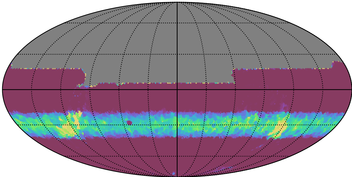
extra_ss_neo2_v3.4_10yrs All sky y band: Min normairmass
