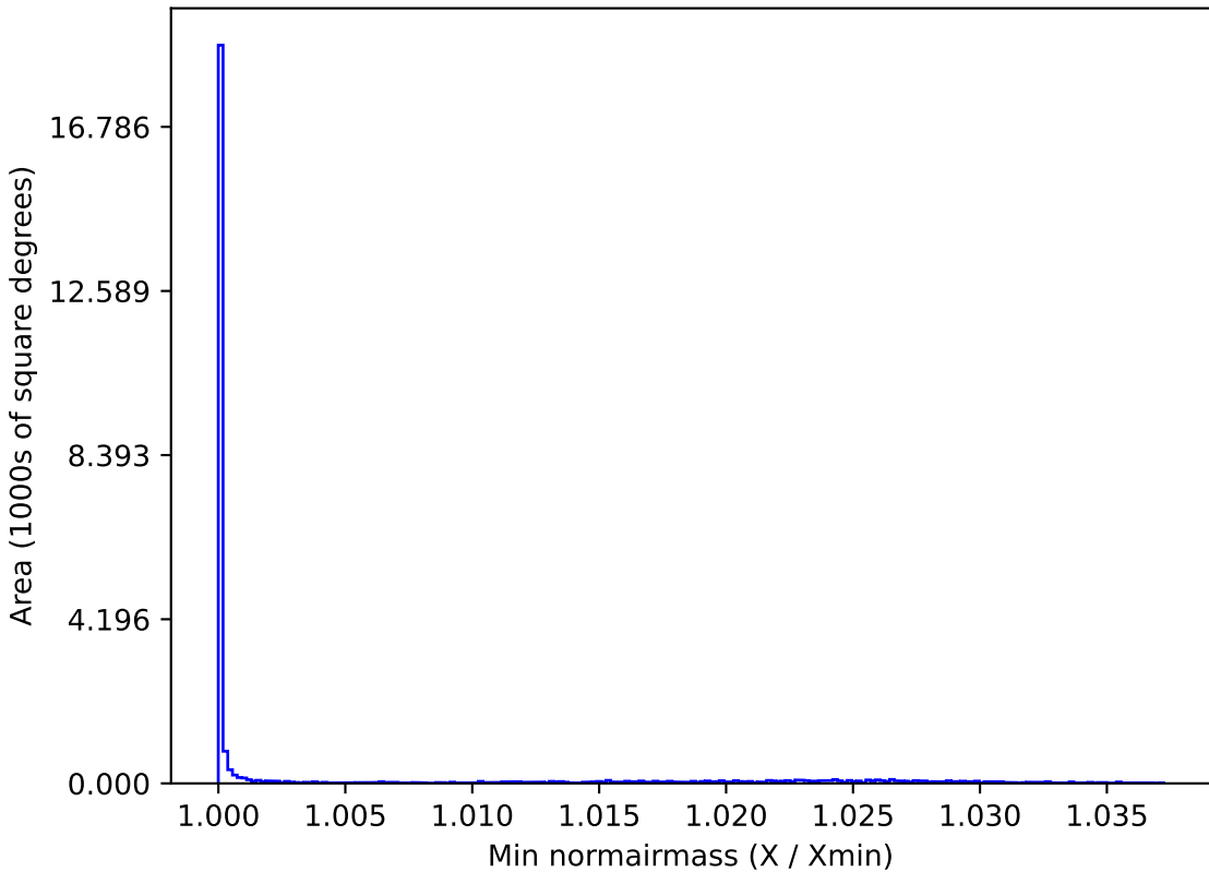
extra_ss_neo2_v3.4_10yrs All sky r band: Min normairmass
