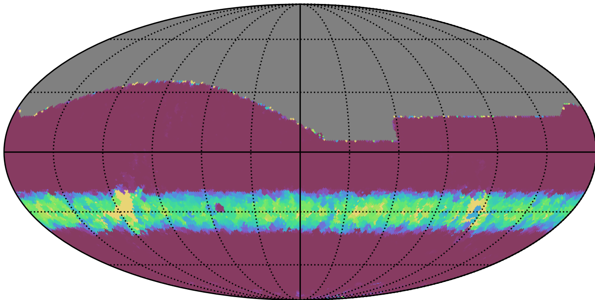
extra_ss_neo2_v3.4_10yrs All sky i band: Min normairmass
