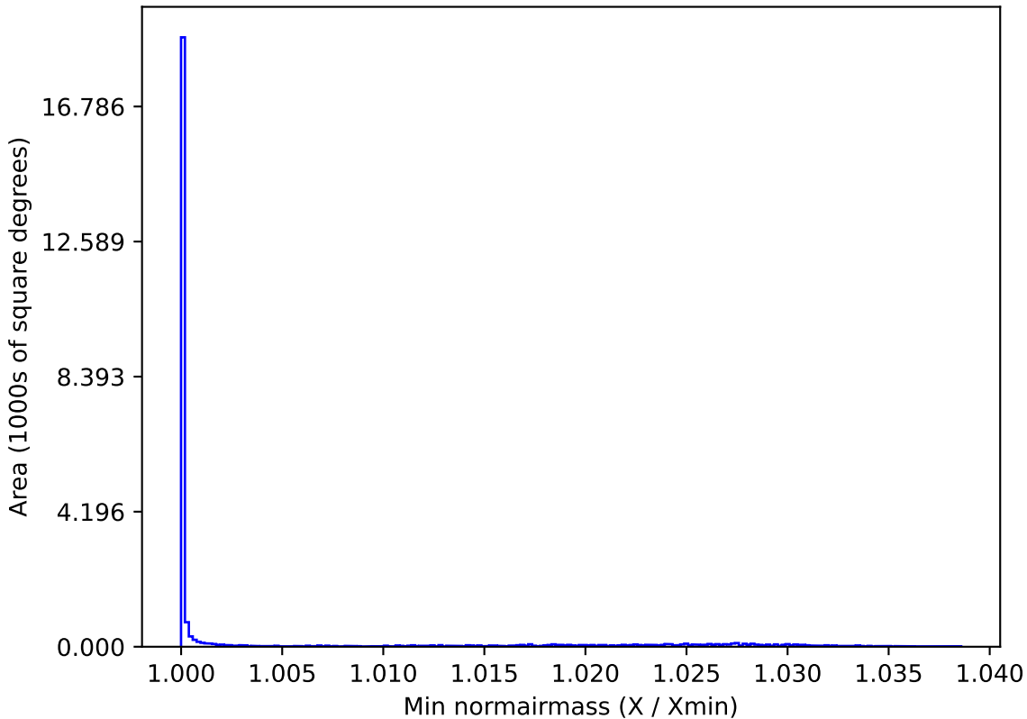
extra_ss_neo2_v3.4_10yrs All sky i band: Min normairmass
