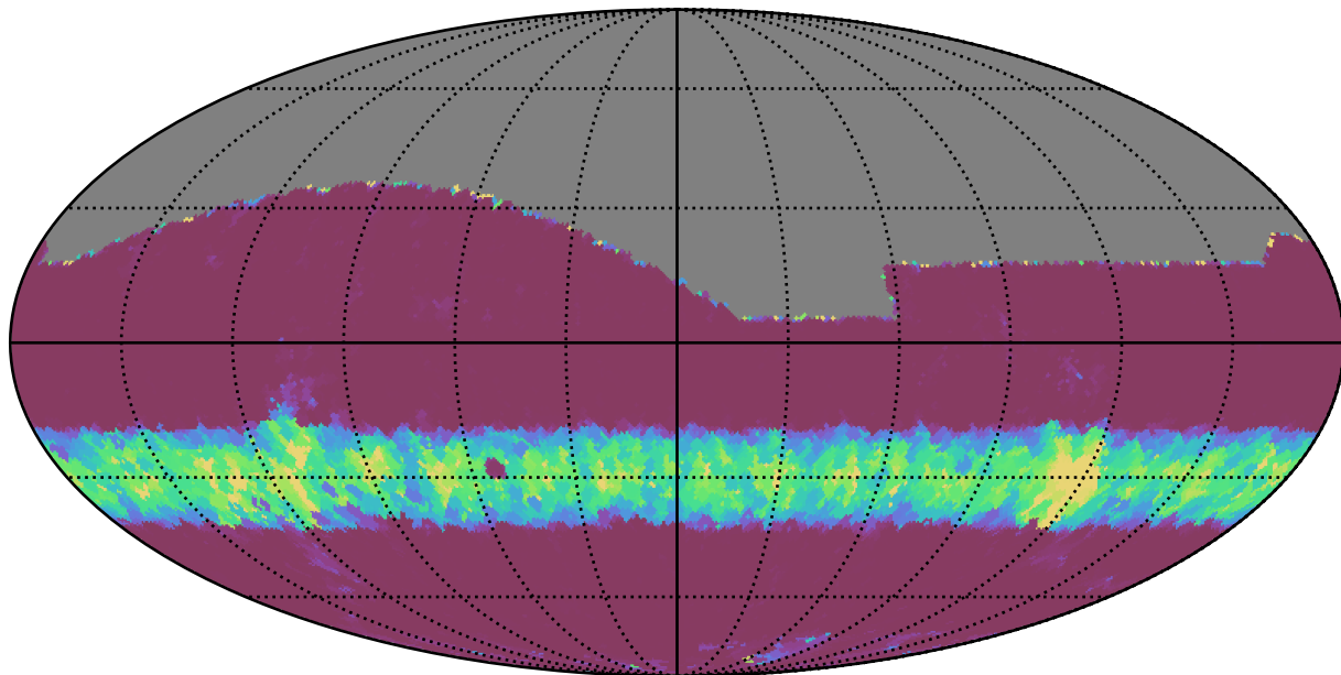
extra_ss_neo2_v3.4_10yrs All sky g band: Min normairmass
