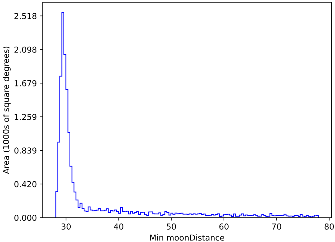
extra_ss_neo2_v3.4_10yrs WFD z band: Min moonDistance
