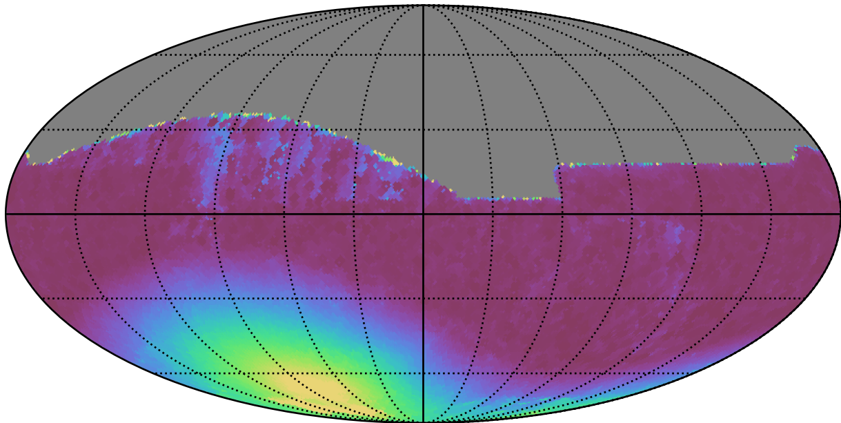
extra_ss_neo2_v3.4_10yrs All sky z band: Min moonDistance
