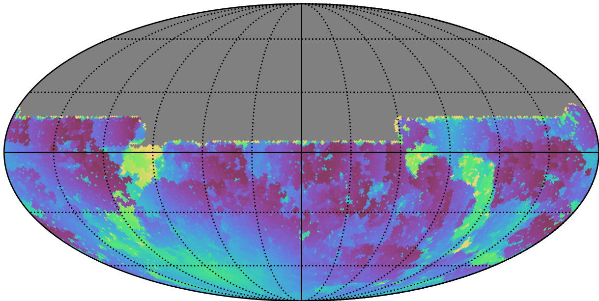
extra_ss_neo2_v3.4_10yrs All sky u band: Min moonDistance
