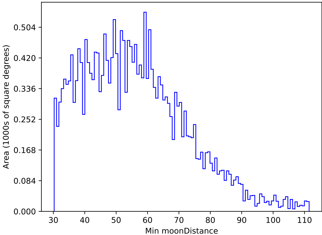
extra_ss_neo2_v3.4_10yrs All sky u band: Min moonDistance
