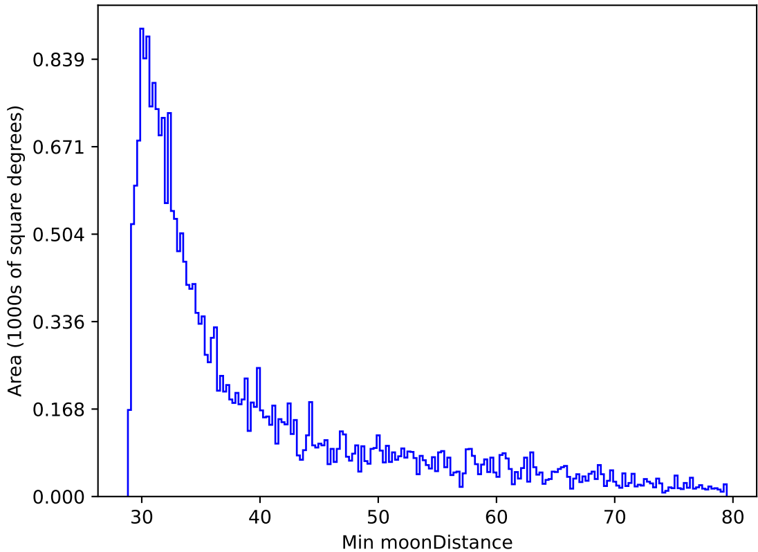
extra_ss_neo2_v3.4_10yrs All sky r band: Min moonDistance
