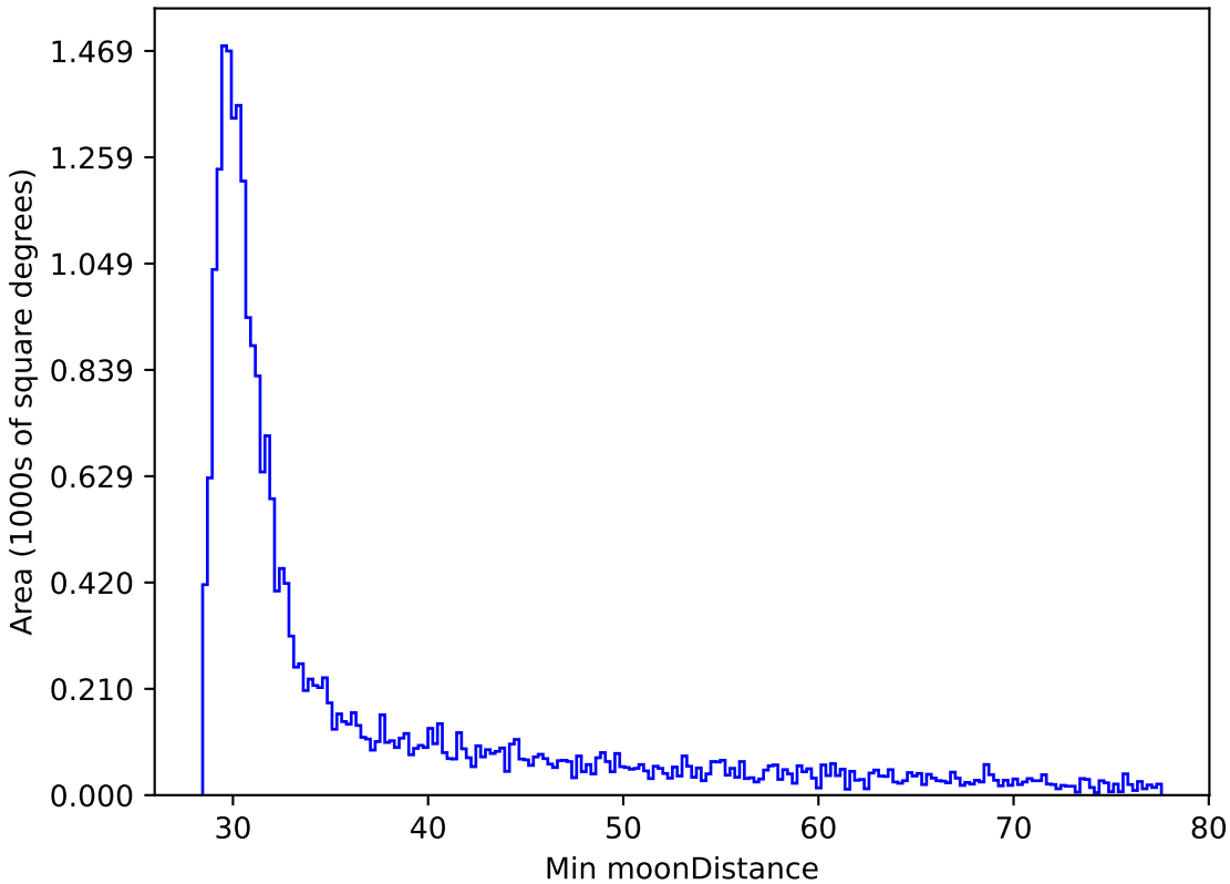
extra_ss_neo2_v3.4_10yrs All sky i band: Min moonDistance
