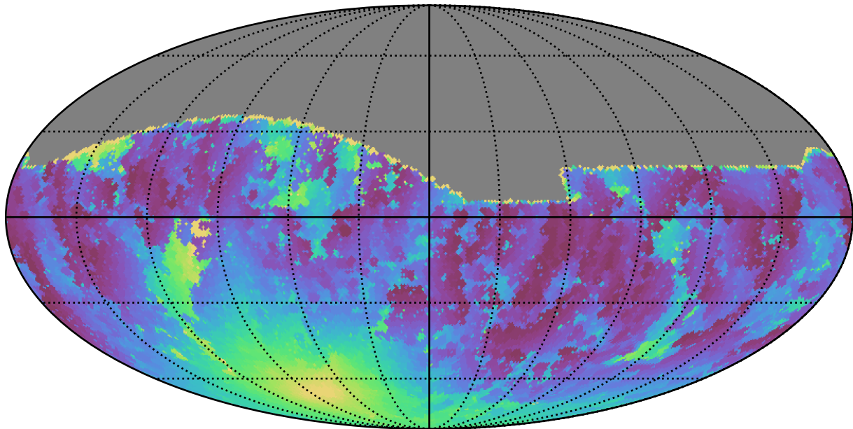
extra_ss_neo2_v3.4_10yrs All sky g band: Min moonDistance
