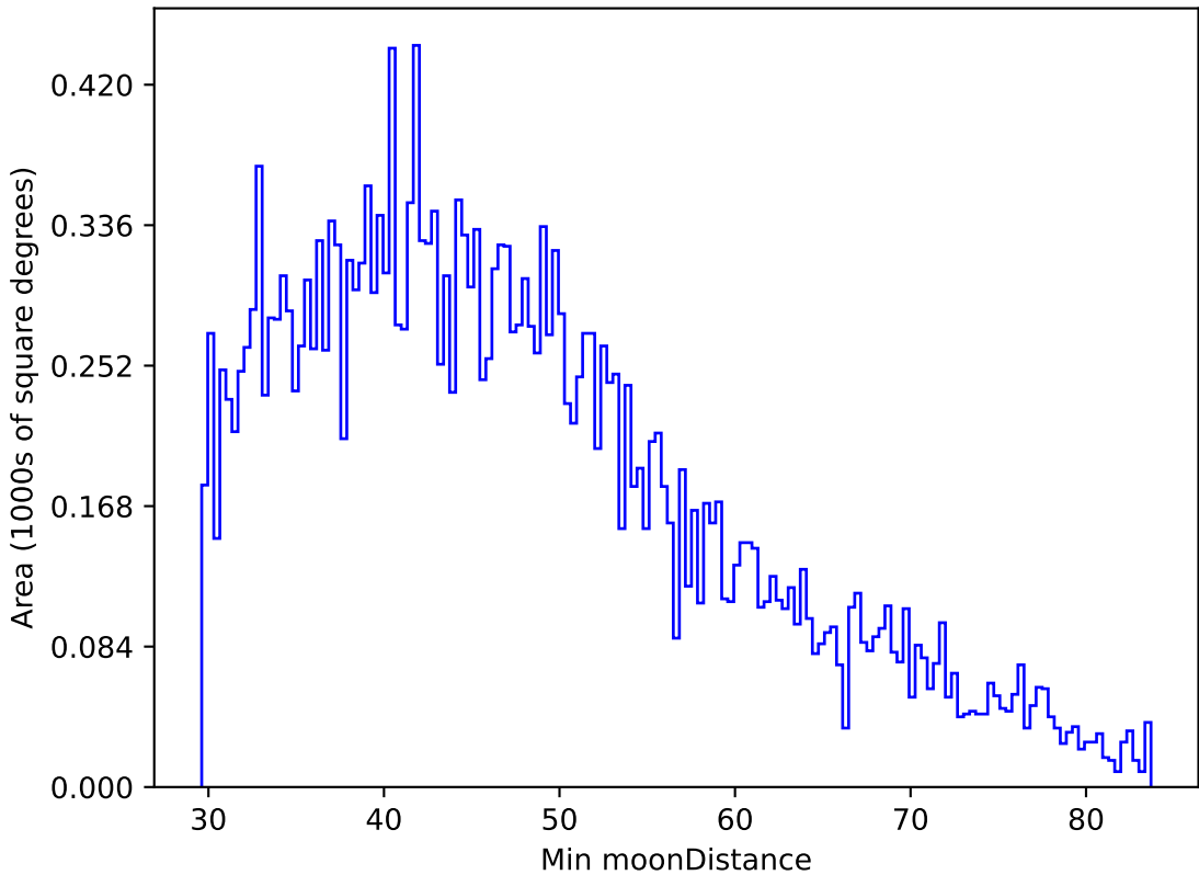
extra_ss_neo2_v3.4_10yrs All sky g band: Min moonDistance
