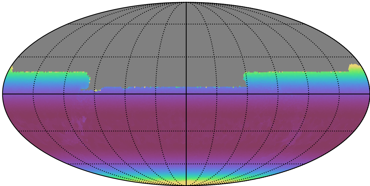
extra_ss_neo2_v3.4_10yrs All sky y band: Min airmass
