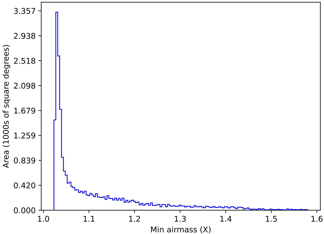
extra_ss_neo2_v3.4_10yrs All sky y band: Min airmass
