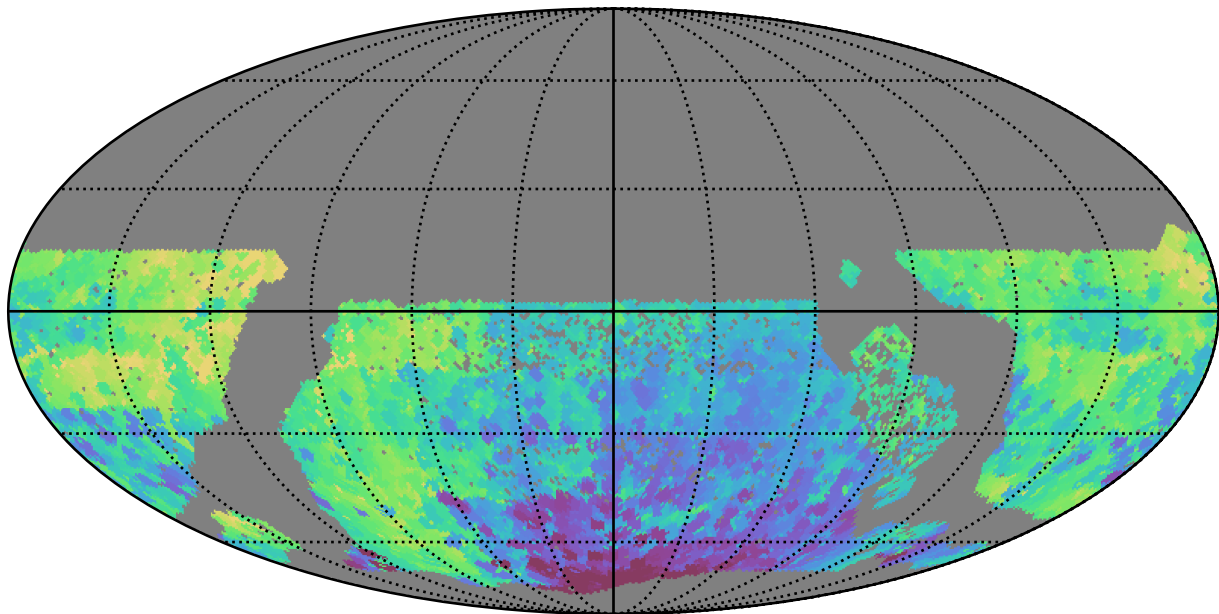
extra_ss_neo2_v3.4_10yrs WFD y band: Min HA
