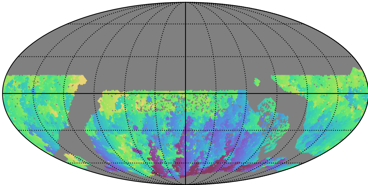
extra_ss_neo2_v3.4_10yrs WFD u band: Min HA
