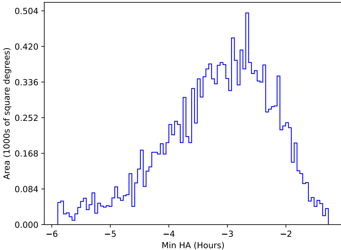
extra_ss_neo2_v3.4_10yrs WFD u band: Min HA
