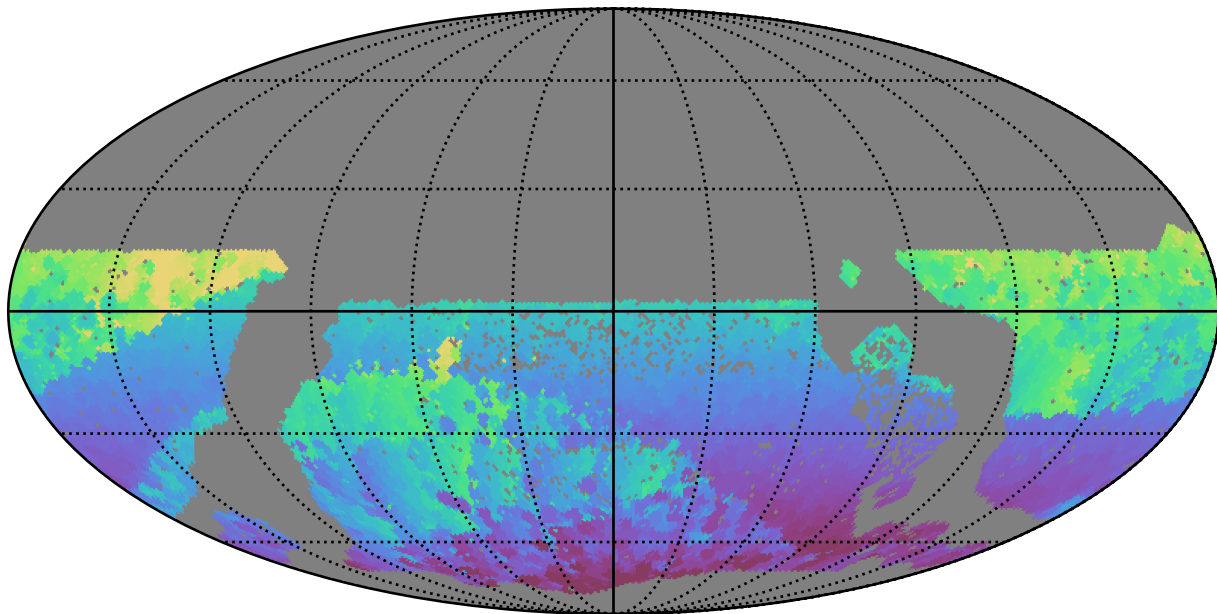
extra_ss_neo2_v3.4_10yrs WFD r band: Min HA
