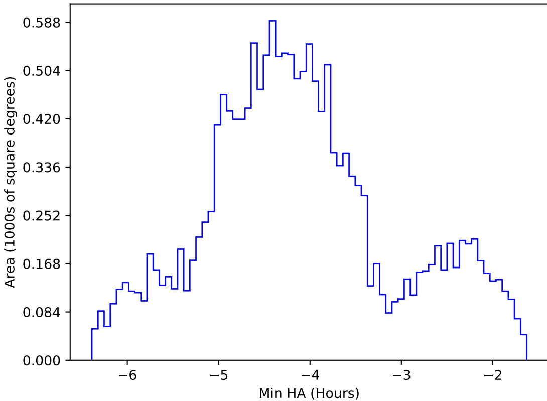
extra_ss_neo2_v3.4_10yrs WFD g band: Min HA
