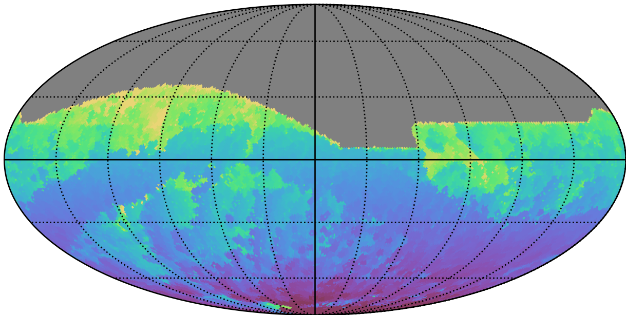
extra_ss_neo2_v3.4_10yrs All sky z band: Min HA
