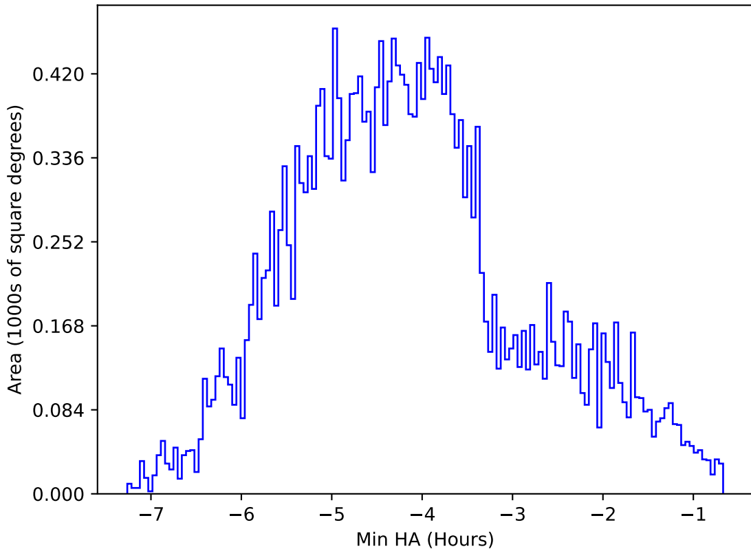
extra_ss_neo2_v3.4_10yrs All sky z band: Min HA
